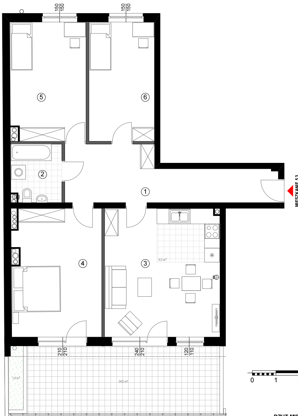
RZUT MIESZKANIA
