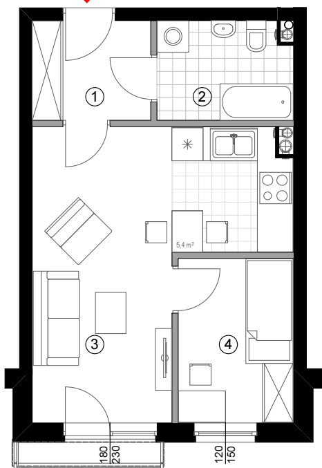
MIESZKANIE 2.2
